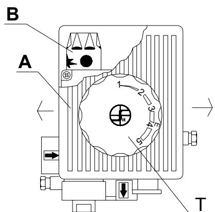
OBRÁZEK 13 OVLÁDACÍ PRVKY
