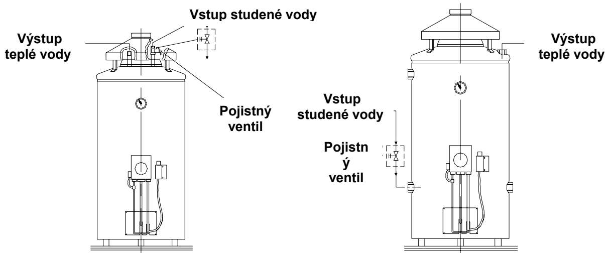
Obrázek 4 Stacionární plynový ohřívač vody pro komerční použití
