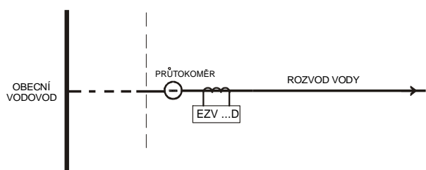
obr. 1 Napojení na obecní vodovod
