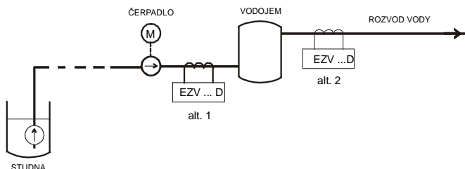
obr. 2 Napojení na vlastní zdroj vody
